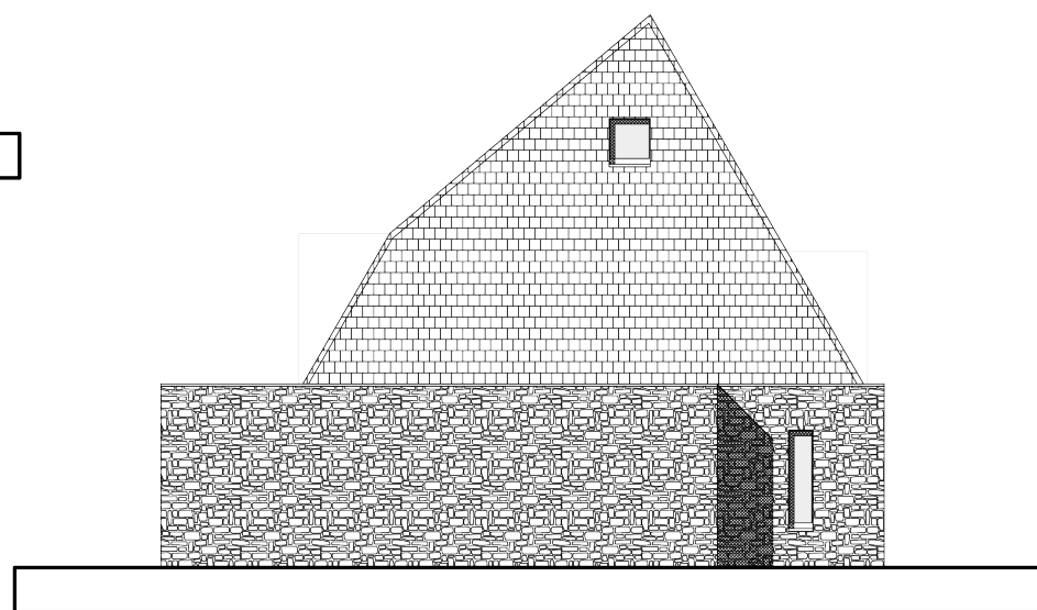
LINKER ZIJGEVEL (oost)
