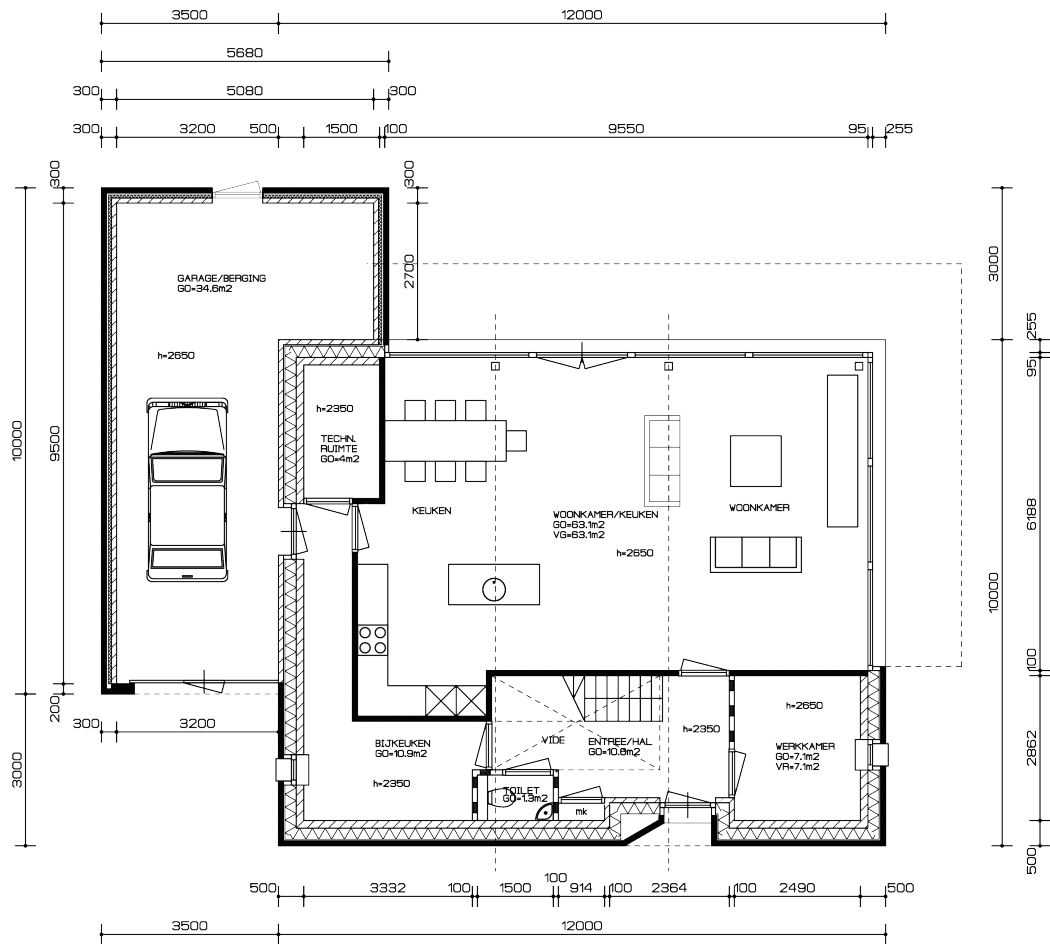
BEGANE GROND
