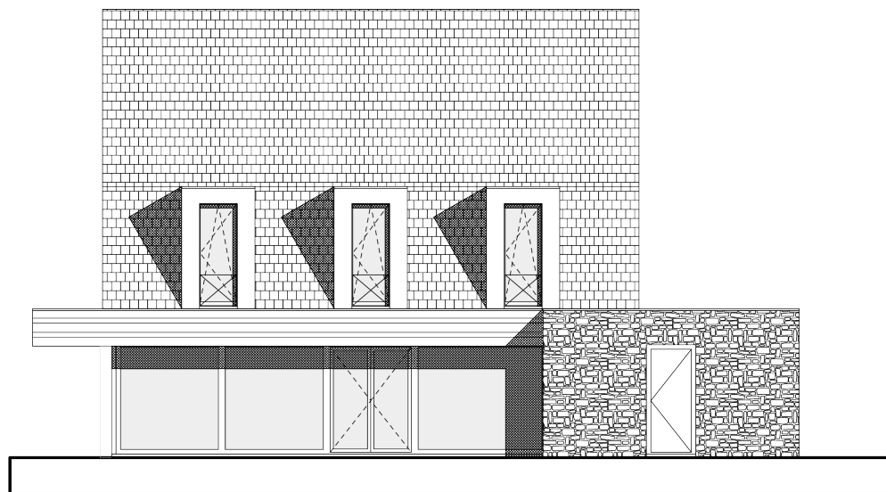
ACHTERGEVEL (zuid)
