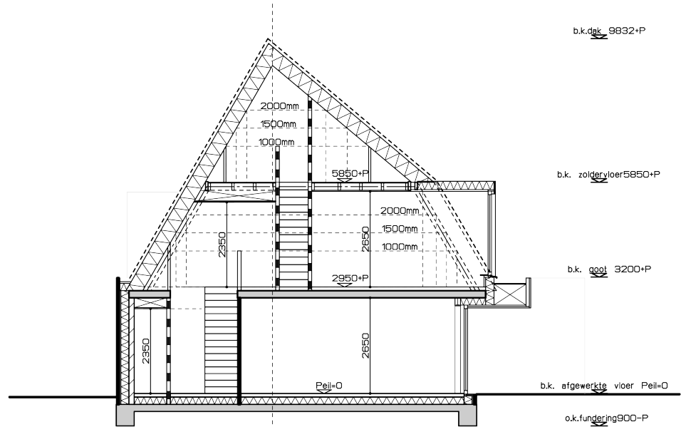
DWARSDOORSNEDE
