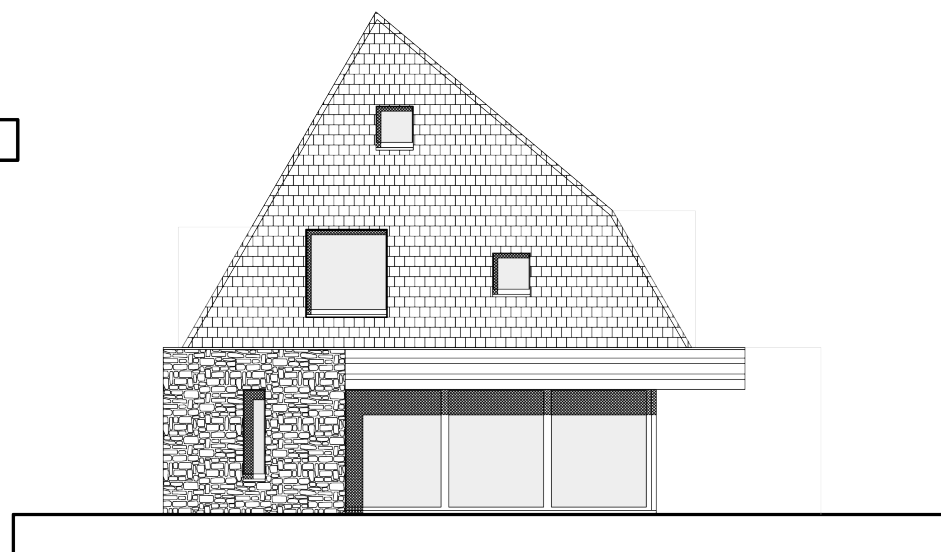
RECHTER ZIJGEVEL (west)
